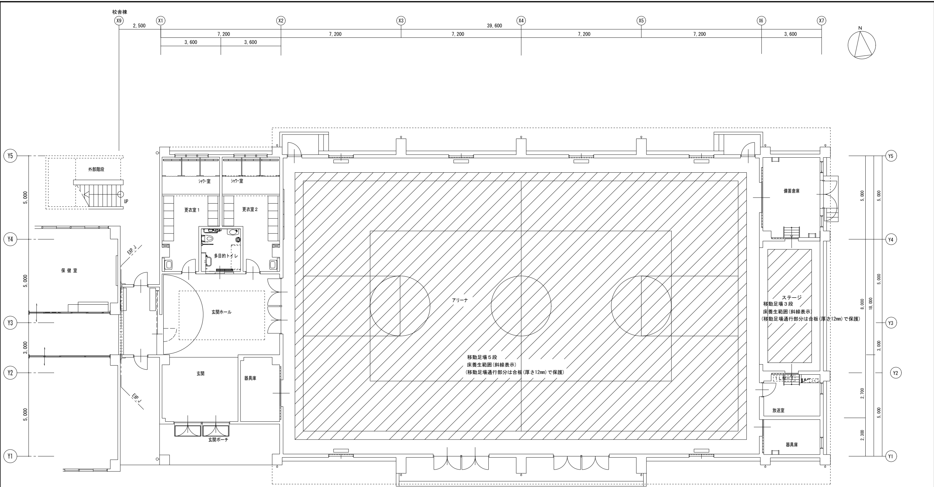
増築屋内運動場棟 1階平面図 S=1/100
