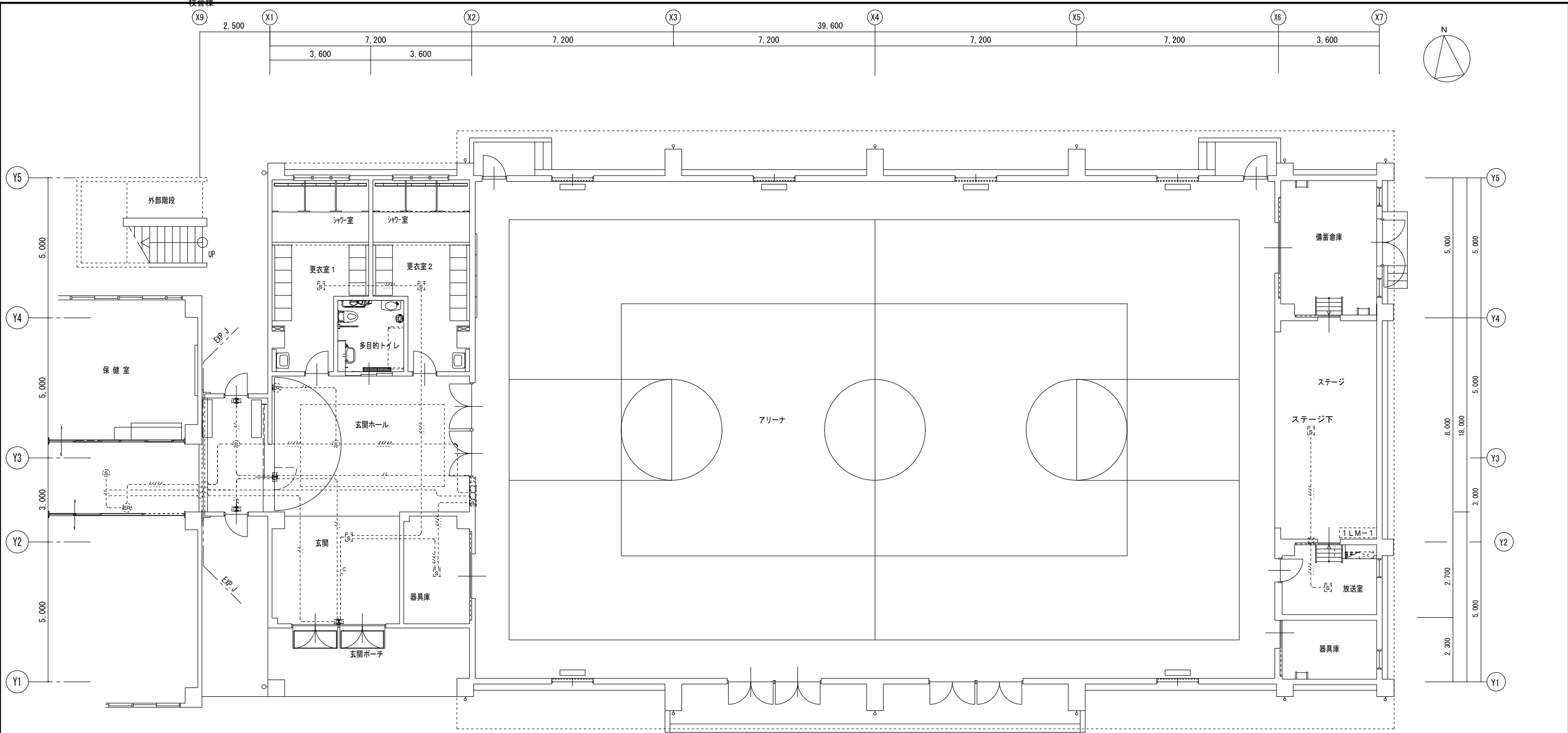
屋内運動場棟 1階平面図 S=1/100
