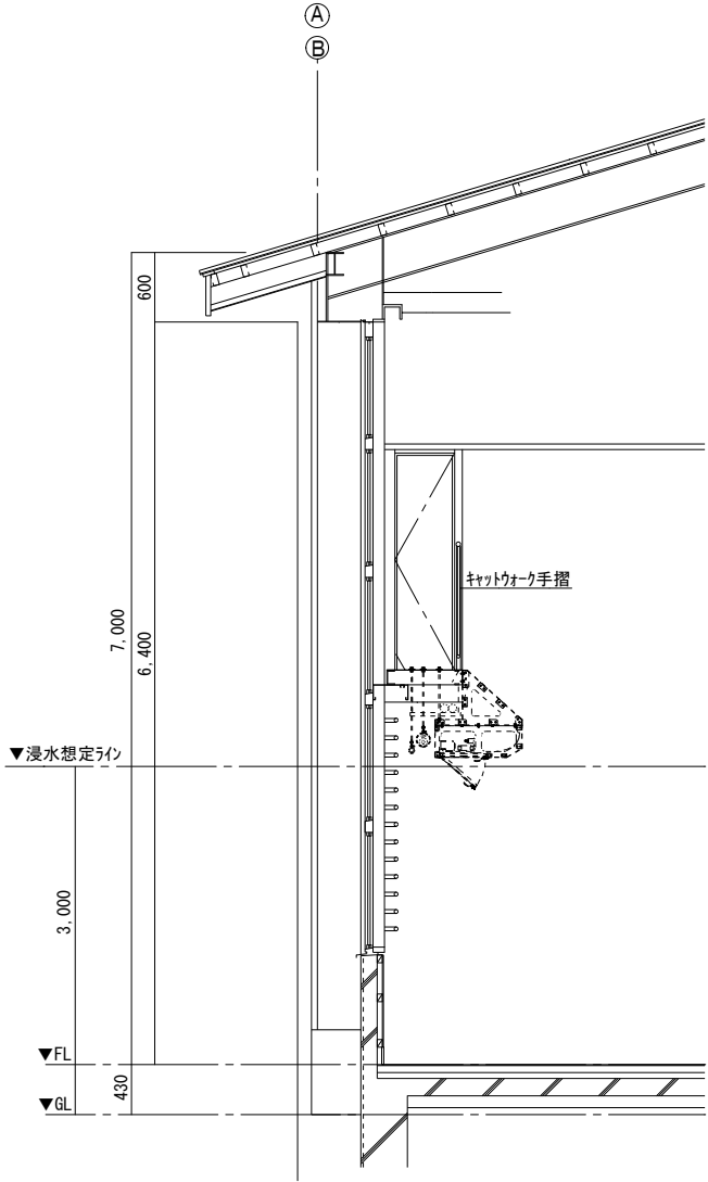
参考断面詳細図 S=1/50
